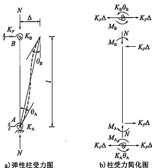
图 E-1 弹性约束柱
