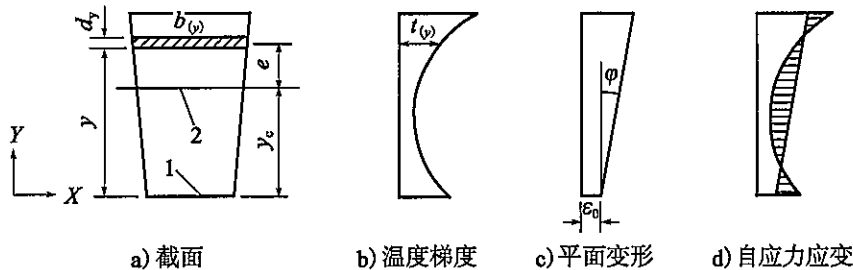
图 D-1 温度梯度计算模式
