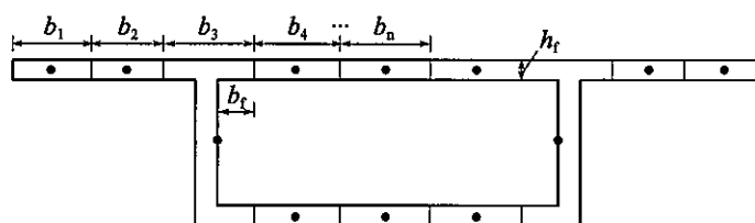
图 A.2.1 空间网格模型示意
