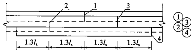
图 9.1.9-2 束筋的搭接
