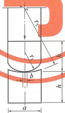
图 8.6.1 混凝土铰
