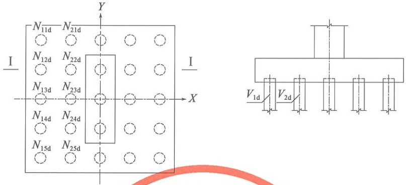
图 8-13 V_d 计算示意
