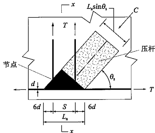
a) 压杆和节点区尺寸示意
