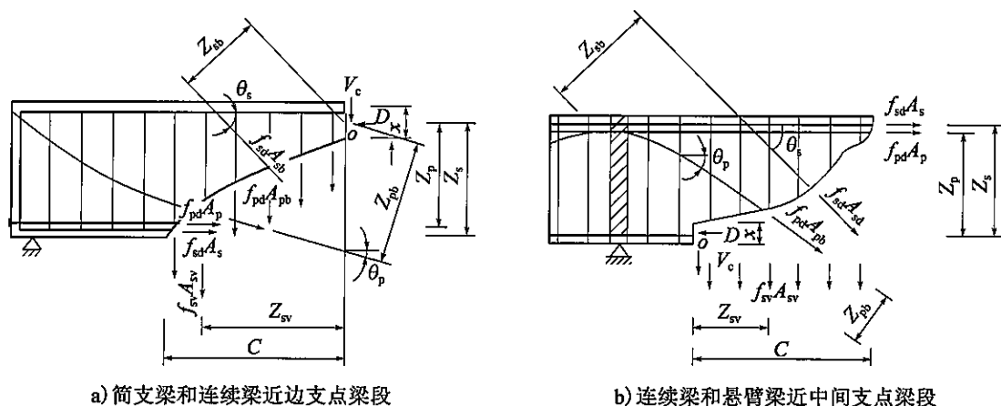
图 5.2.9 斜截面抗剪承载力验算
