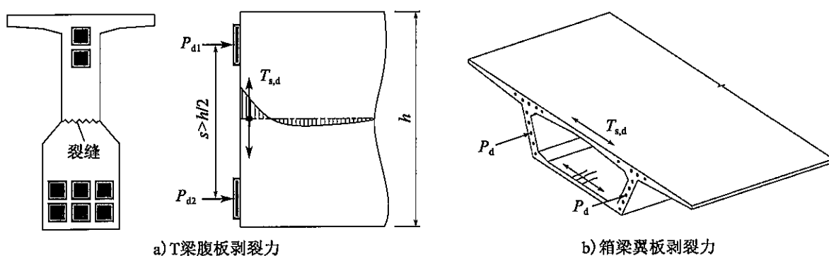
图 8-7 大间距锚头间的剥裂力及可能产生的裂缝
