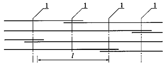
图 9.1.9-1 受力钢筋绑扎接头
