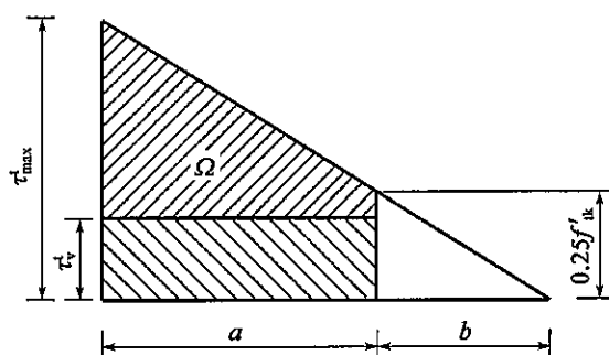
图 7.2.6 钢筋混凝土受弯构件剪应力分配 a-箍筋、弯起钢筋承受剪应力的区段;b-混凝土承受剪应力的区段
