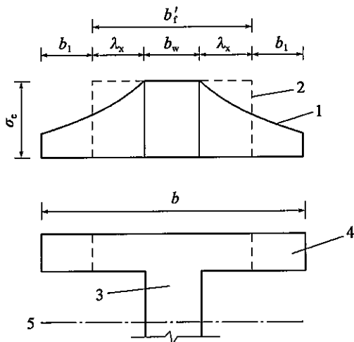
图 4-8 T 形截面梁应力示意
