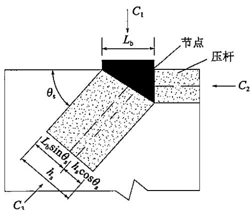
图 B.3.3-1 集中力下的压杆和 CCC 节点区
