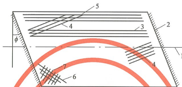
图 9.2.6 斜板桥钢筋布置
