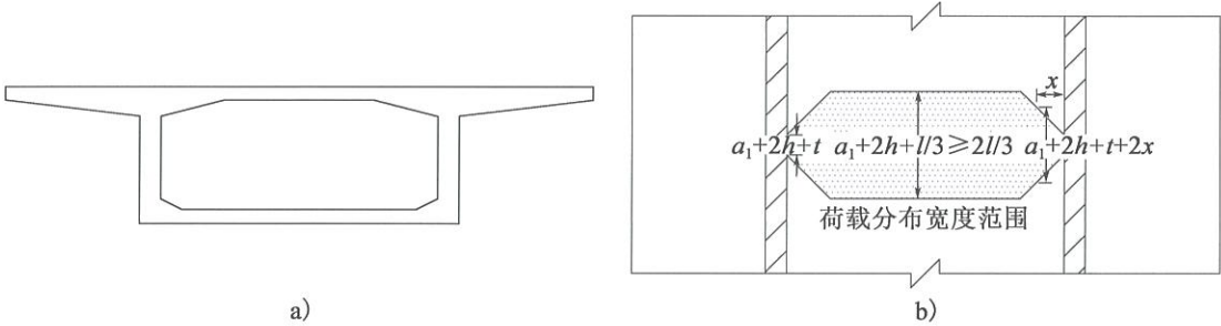
图 4-6 轮载分布宽度计算示意
