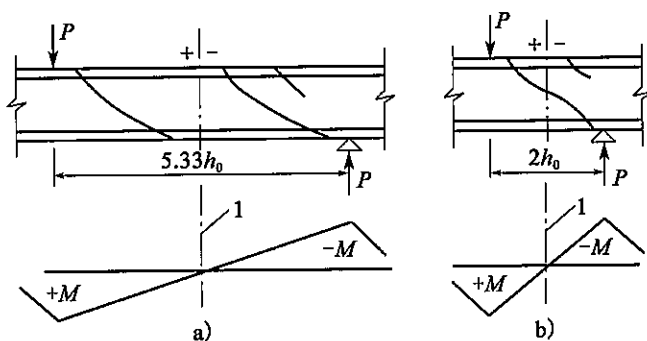
图 5-3 承受异号弯矩钢筋混凝土梁的典型剪切破坏
