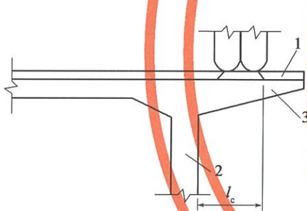
图 4.2.5 车轮荷载在悬臂板上的分布 1-桥面铺装;2-腹板;3-悬臂板
