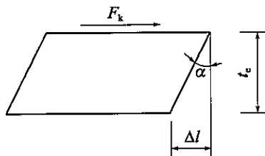
图 8-16 支座橡胶层剪切变形
