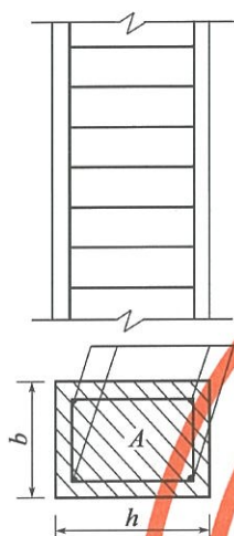
图 5.3.1 配有箍筋的钢筋混凝土轴心受压构件
