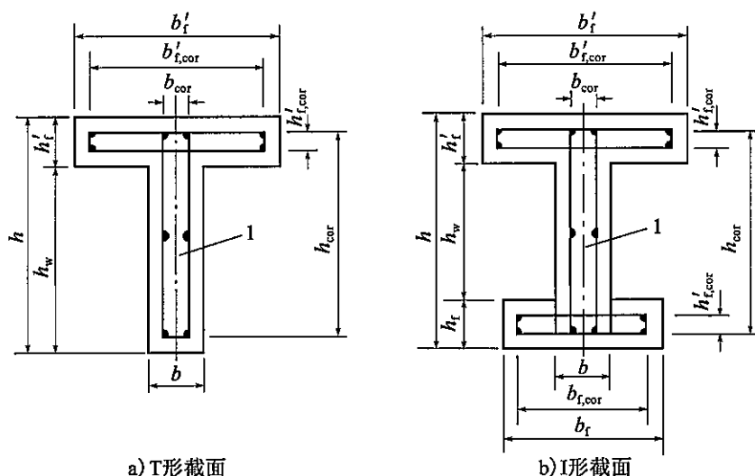
图 5.5.5 T形和I形受扭构件截面
