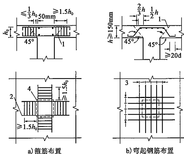
图 9.2.9 独立墩柱顶面抗冲击钢筋配置
