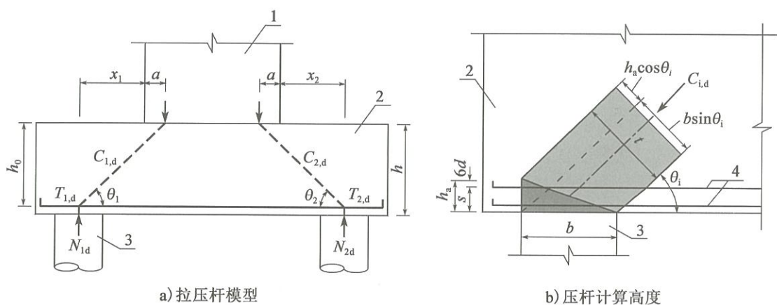
图 8.5.4 承台按拉压杆模型计算
