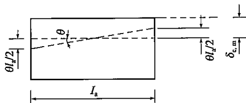
图 8-17 支座的压缩变形
