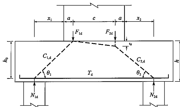
图 8-15 带倾角水平压杆的拉压杆模型
