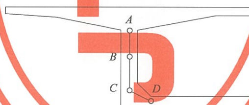
图 A-3 箱梁应力计算位置示意
