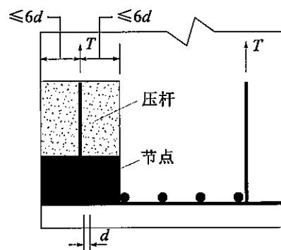
图 B.3.3-2 由钢筋和支承约束形成的压杆和 CCT 节点区
