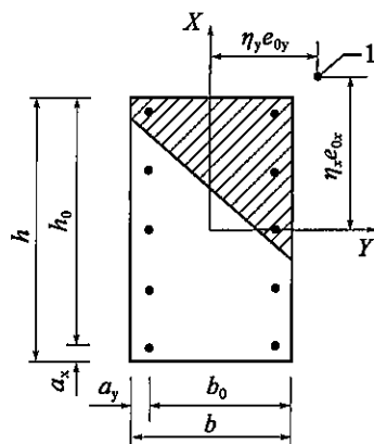
图 5.3.11 钢筋混凝土双向偏心受压构件 1-轴向力作用点
